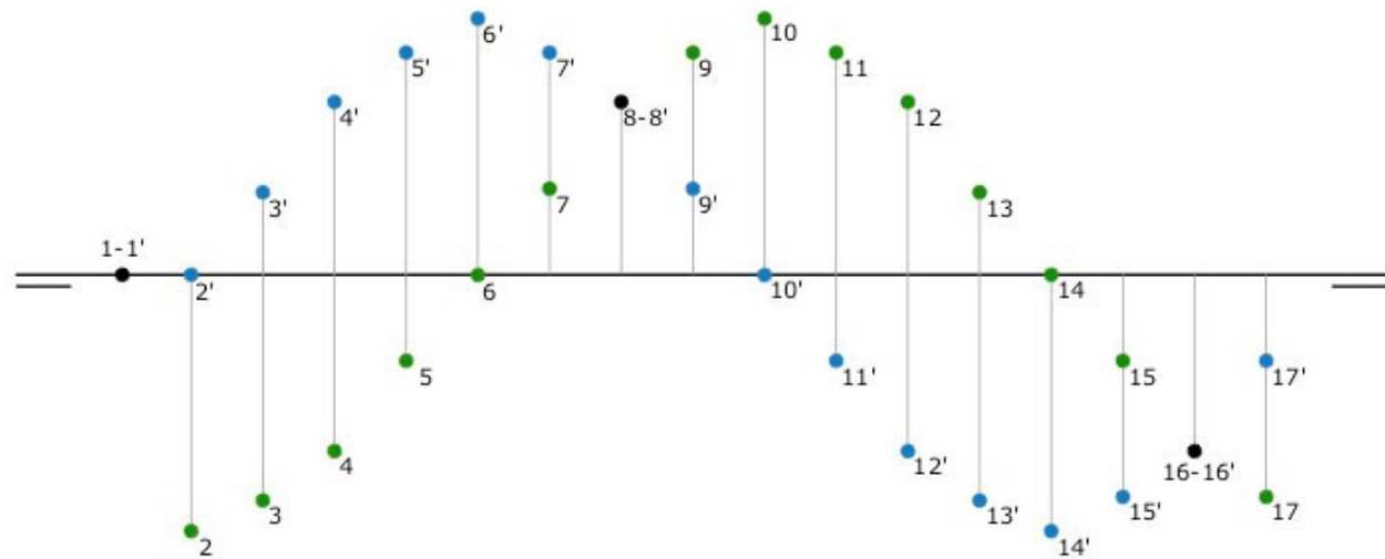
SISTEMA DIÉDRICO
